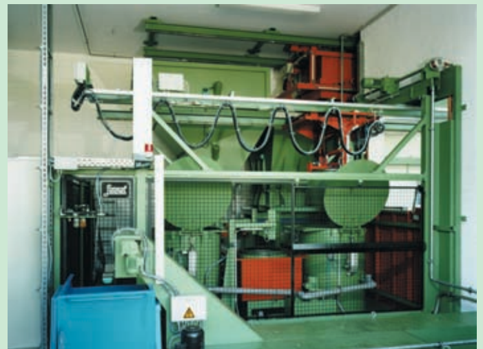
Tratamiento de virutas con un molino de virutas y separación de los diferentes tipos de material.
